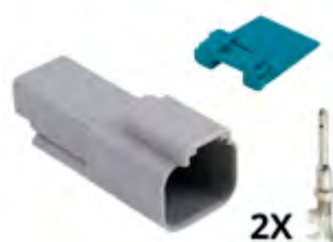
Conector DT04-2P Macho - 2 vias Cód. 1217021
